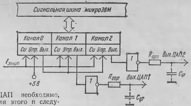
Преобразователь код-аналог на базе БИС КР580ВИ53
