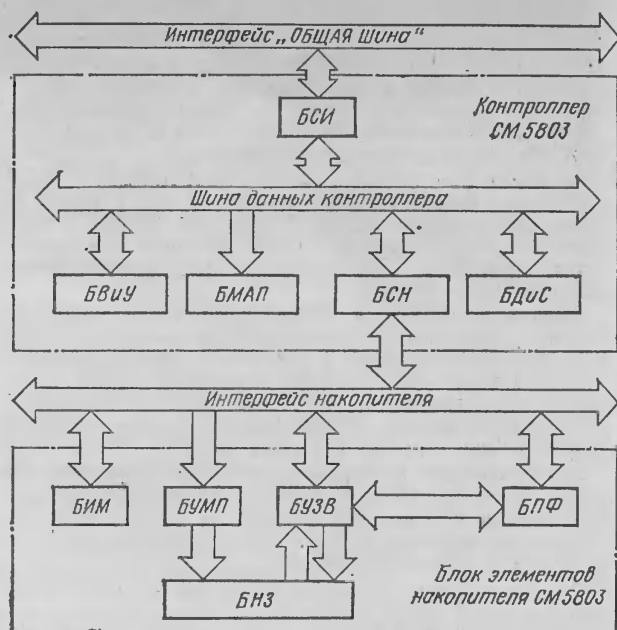
Рис. 1. Структурная схема ЦМД ЗУ СМ 5803
