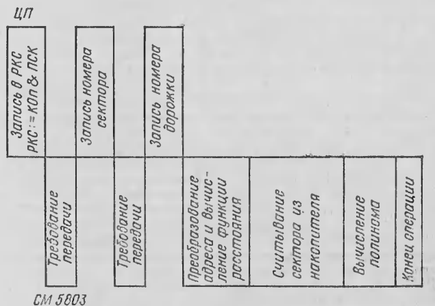
Рис. 4. Диаграмма взаимодействия ЦП и СМ 5803 в режиме чтения
