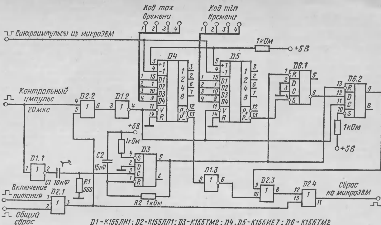
Принципиальная схема устройства контроля времени выполнения программы
