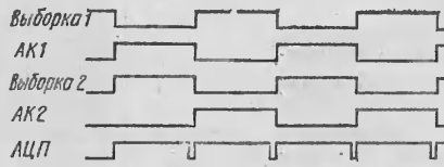
Рис. 2. Временные диаграммы управляющих сигналов
