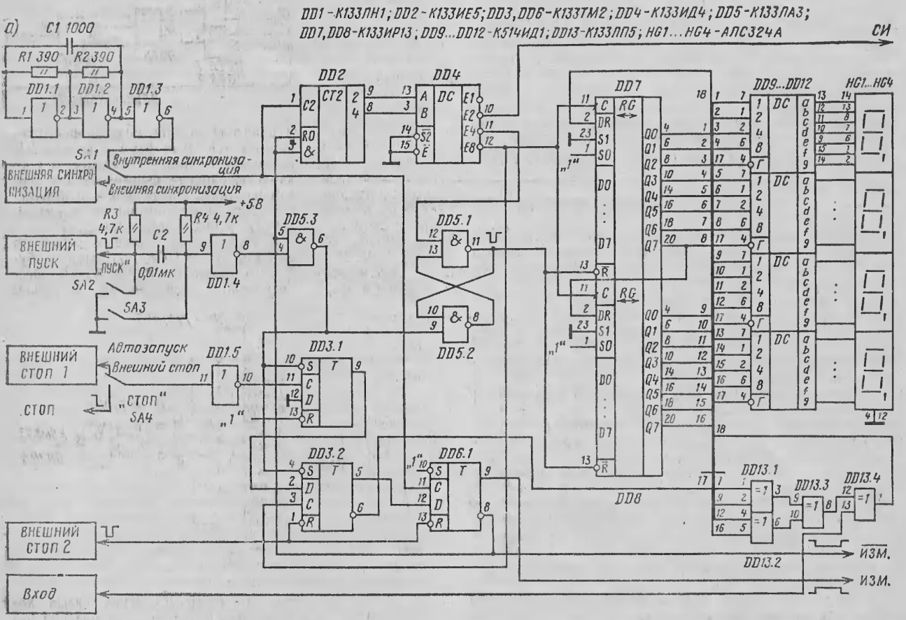
Рис. 1. Принципиальная схема сигнатурного анализатора
