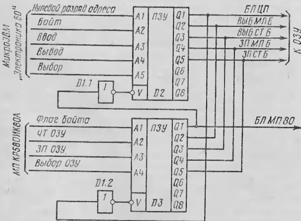
Принципиальная схема разрешения конфликтной ситуации
