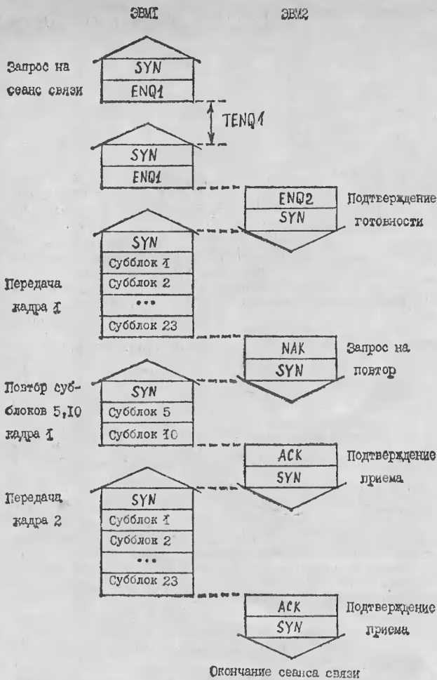
Рис. 3. Процедура передачи двух информационных кадров
