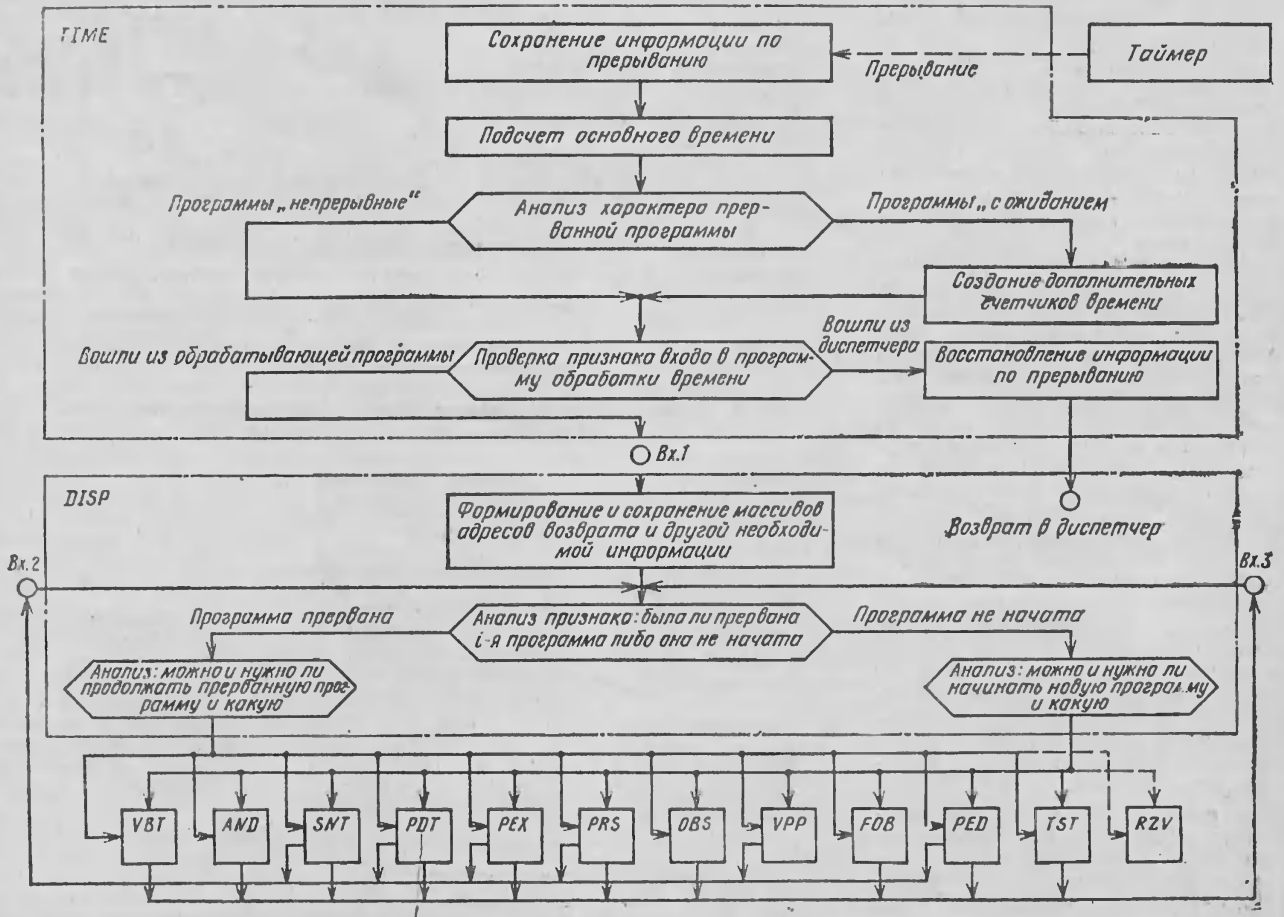
Рис. 4. Функционирование программного обеспечения
