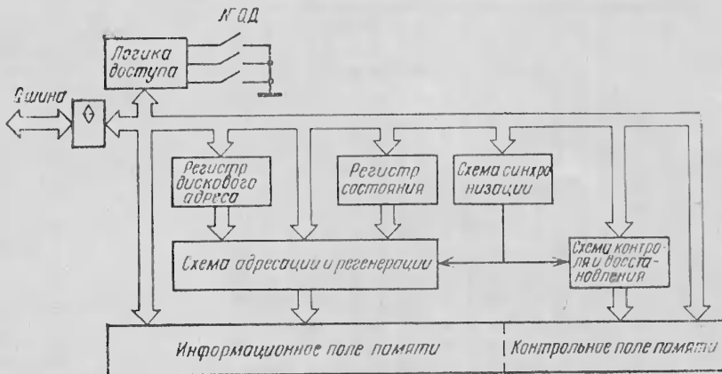
Блок-схема одноплатного электронного диска,
