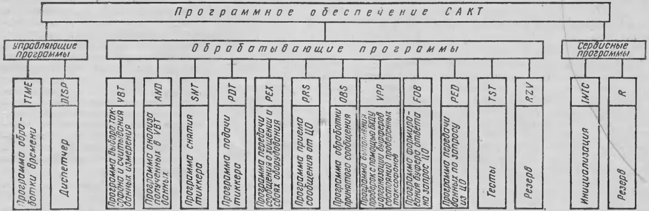
Рис. 3. Состав программного обеспечения системы контроля таксофонов
