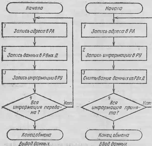
Рис. 2. Блок-схема алгоритмов обмена
