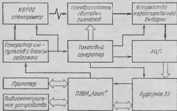
Структурно-функциональная схема ОМА
