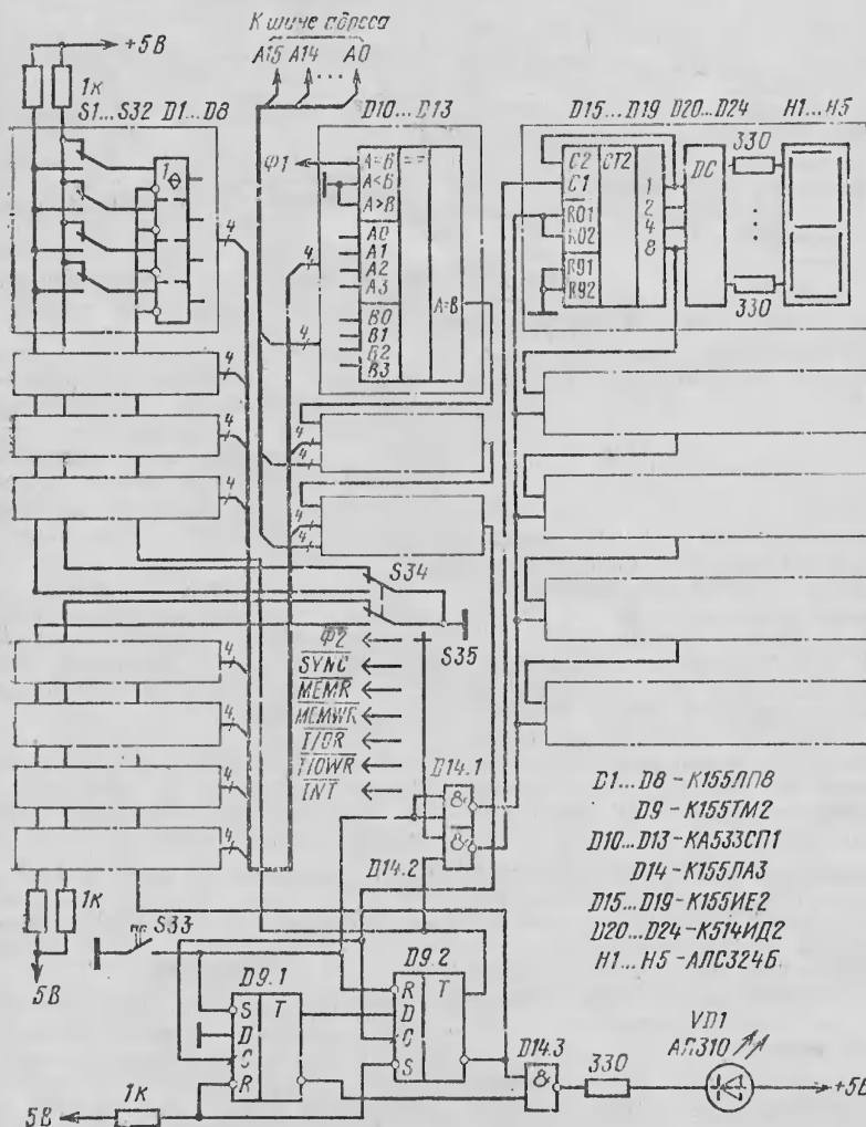
Счетчик сигналов для микропроцессора КР580ВМ80А
