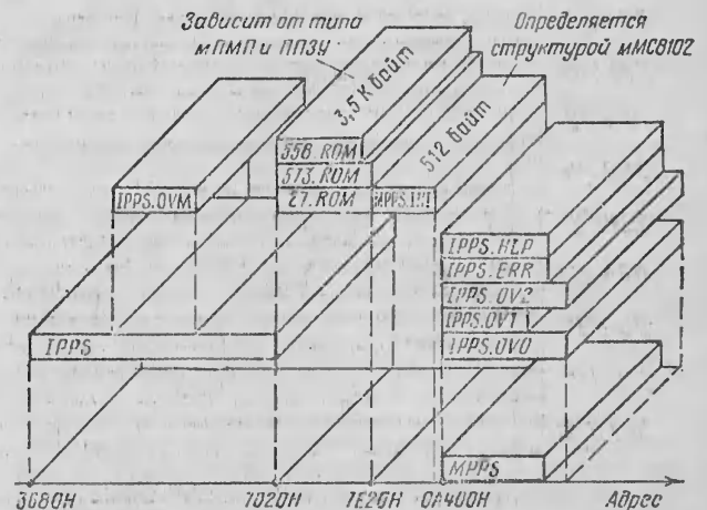
Рис. 1. Организация перекрытий в MPPS
