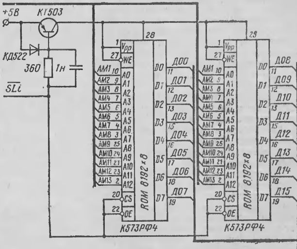
Рис. 3. Схема ячейки ПЗУ-диска
