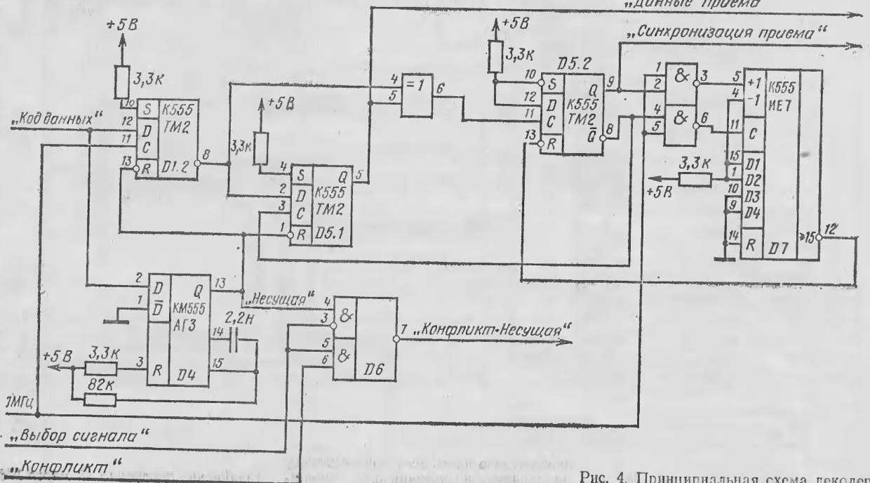
Рис. 4. Принципиальная схема декодера
