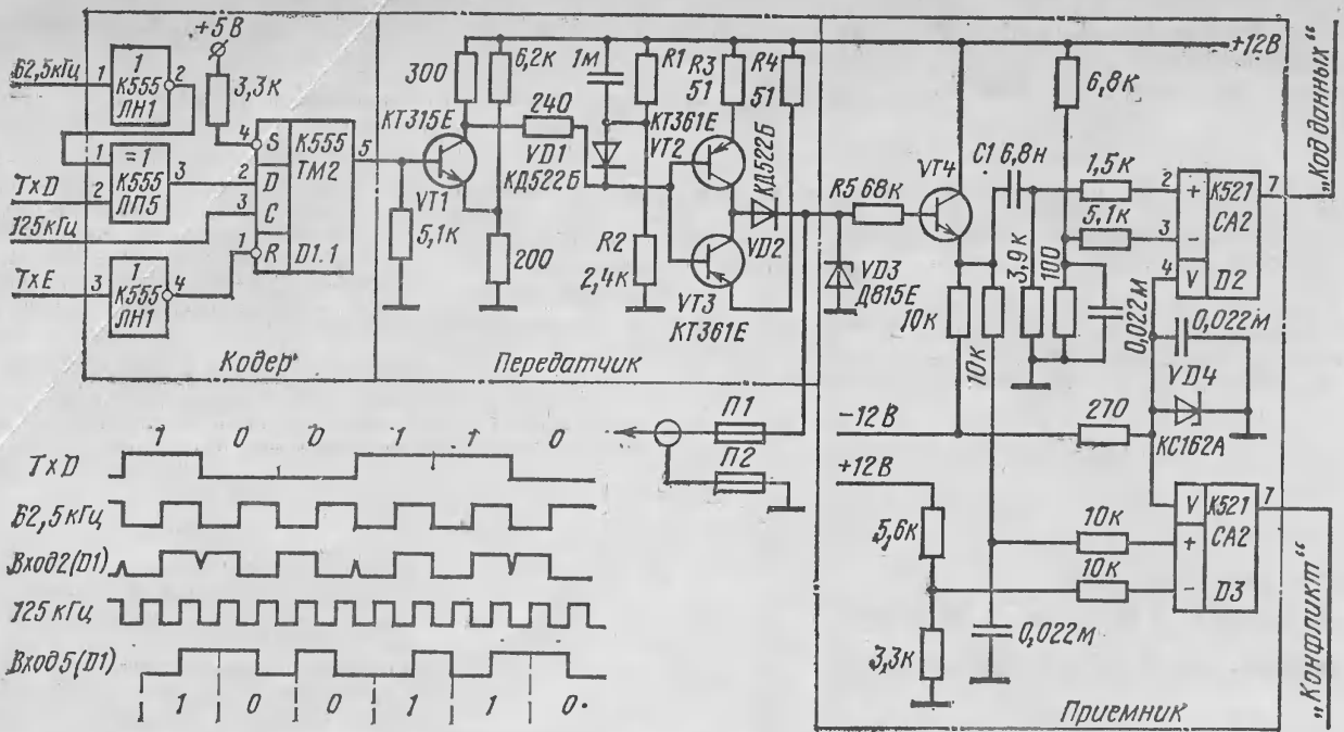
Рис. 2. Принципиальная схема кодера и преопередатчика
