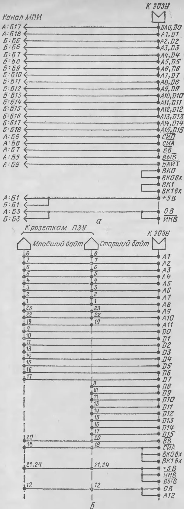
Рис. 2. Схема адаптера для подключения ОЗУ к каналу МПИ (а) и микроконтроллеру (б)
