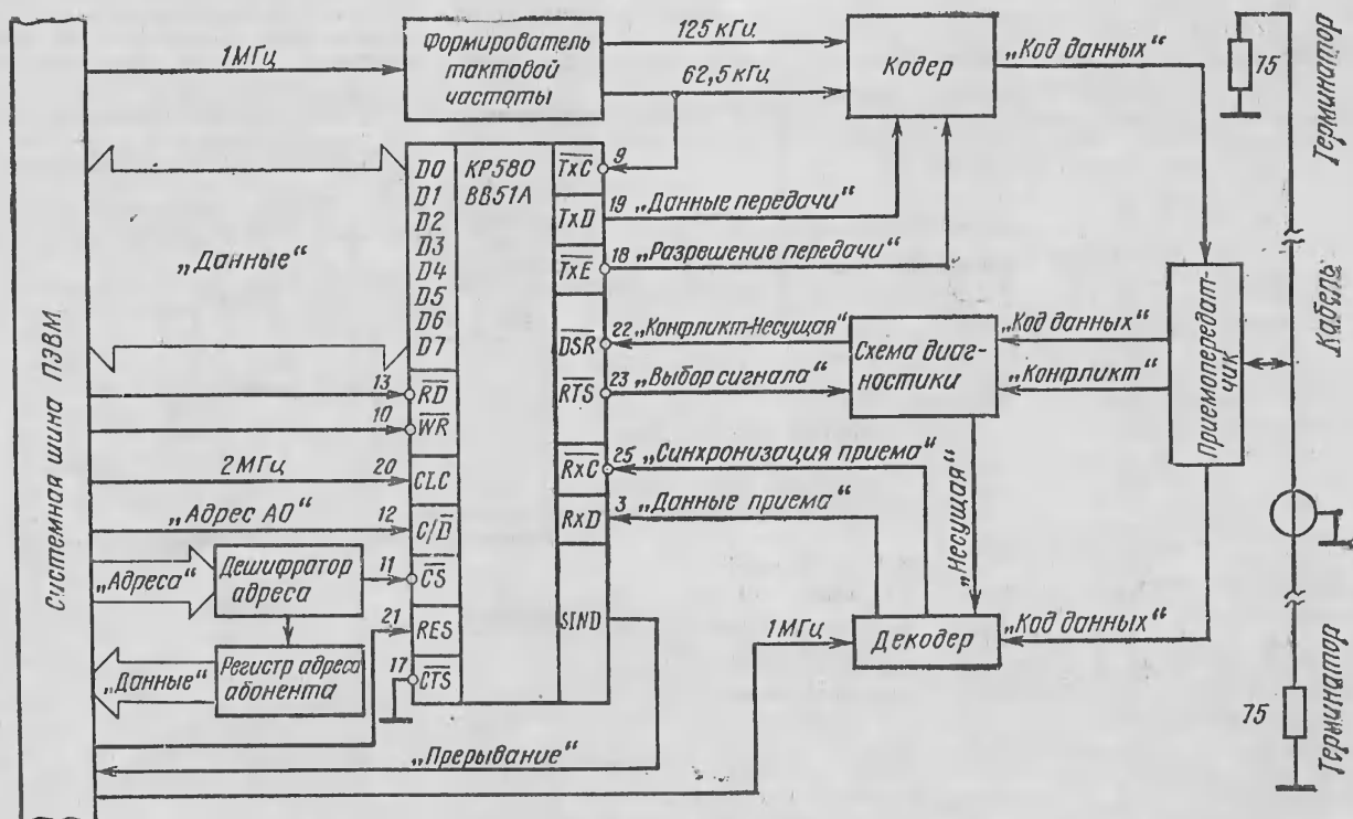
Рис. 1. Функциональная схема УСАПП
