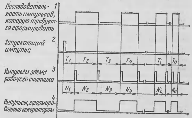
Рис. 1. Принцип формирования импульсов с заданными временными параметрами
