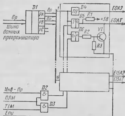
Рис. 2. Функциональная схема ключей адреса
