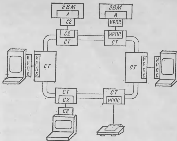
Рис. 1. Структурная схема станции СЛК-СМ
