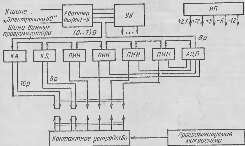
Рис. 1. Структурная схема устройства программирования
