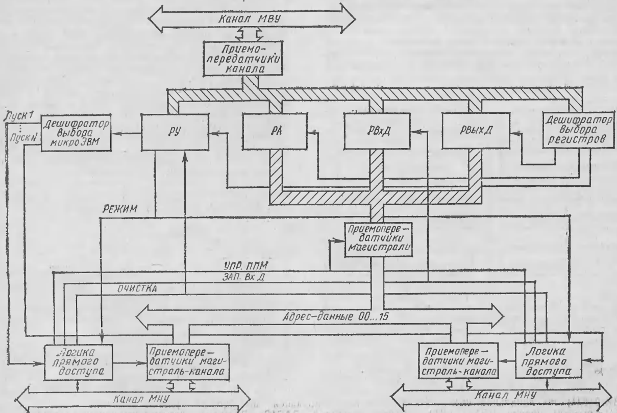
Рис. 1. Структурная схема устройства связи
