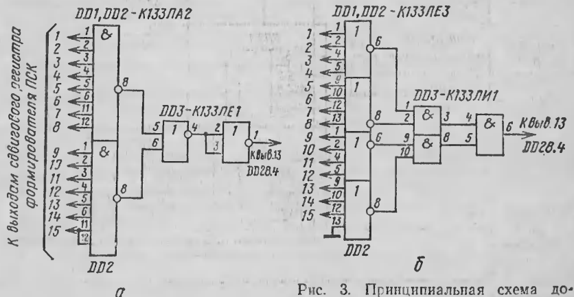
Рис. 3. Принципиальная схема дополнительного узла для сигнатурного анализатора
