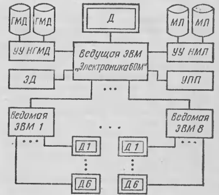
Структура локальной вычислительной сети:
