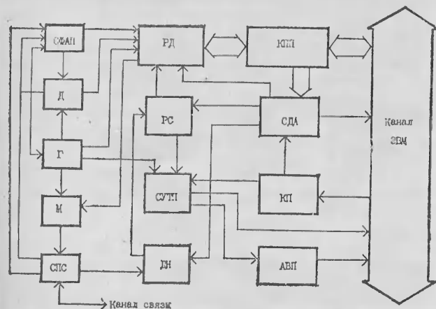
Рис. 1. Блок-схема программно управляемого модема
