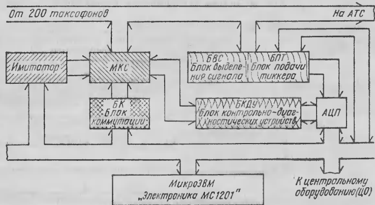
Рис. 1. Структура периферийного оборудования системы автоматизированного контроля таксофонов
