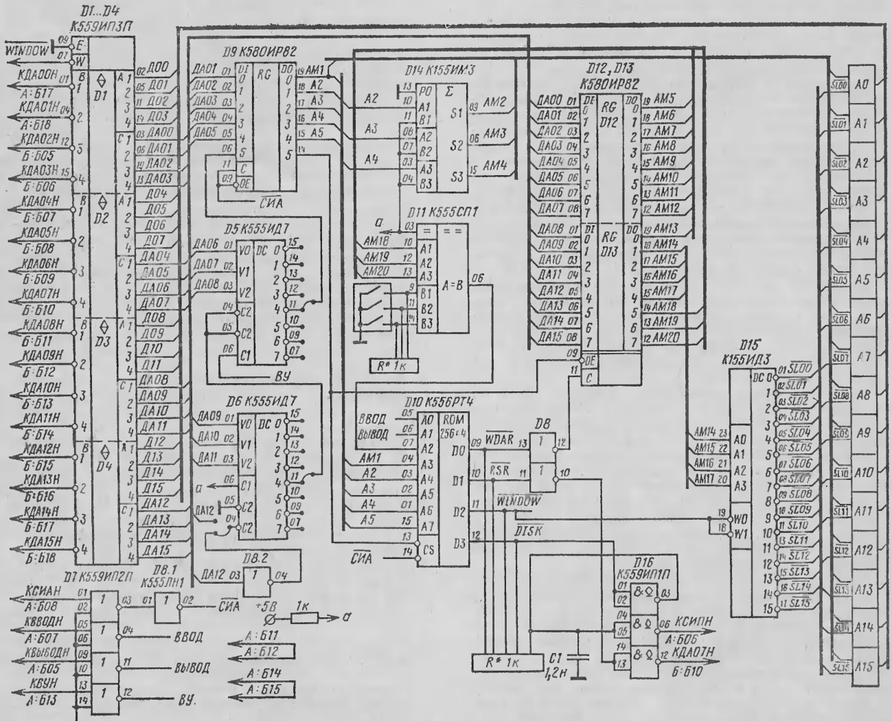
Рис. 1. Схема электронного ПЗУ-диска
