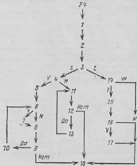
Реализованный алгоритм замены группы символов:
