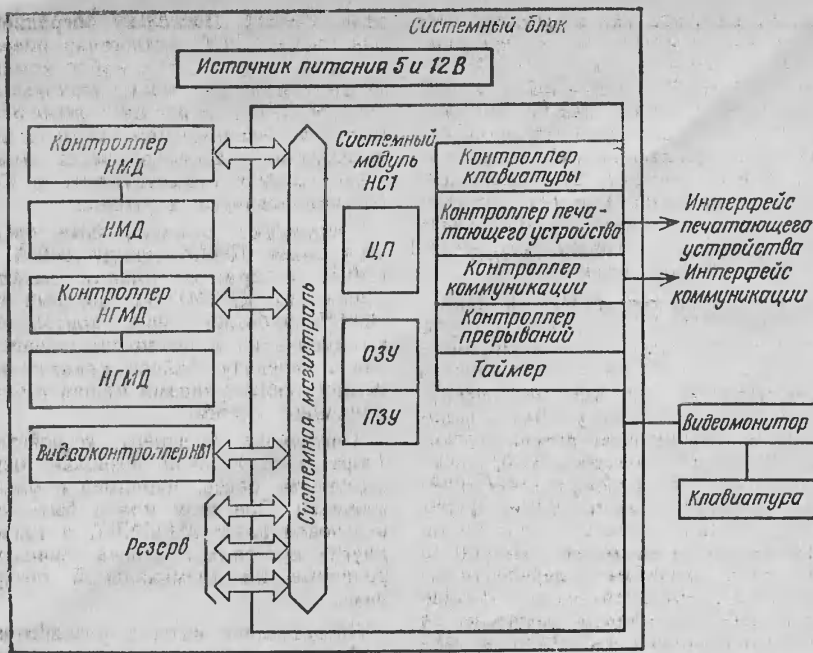
Структурная схема ПЭВМ «Электроника МС 0585»
