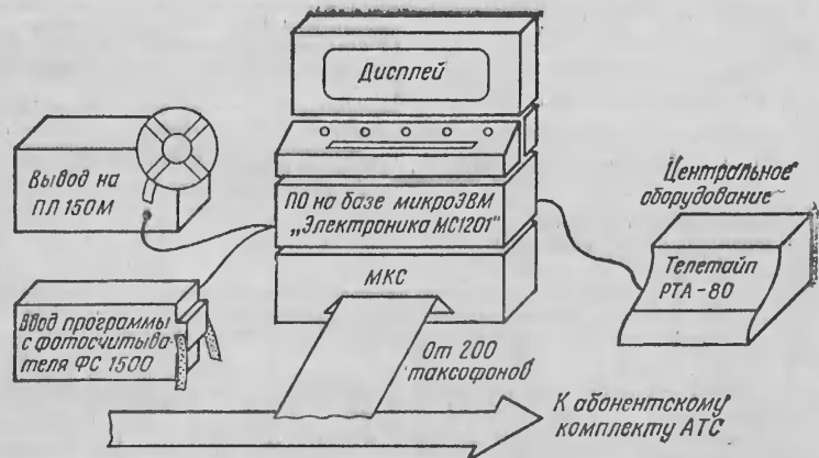
Рис. 2. Состав периферийного оборудования и стенда для отладки программ
