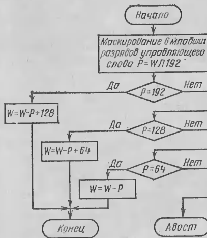
Рис. 3. Блок-схема обработки прерываний при переполнении разрядной сетки
