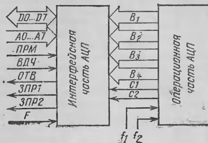
Рис. 1. Структурная схема АЦП
