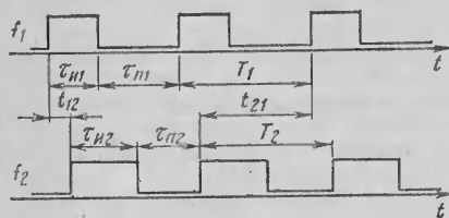
Рис. 2. Параметры преобразуемых сигналов
