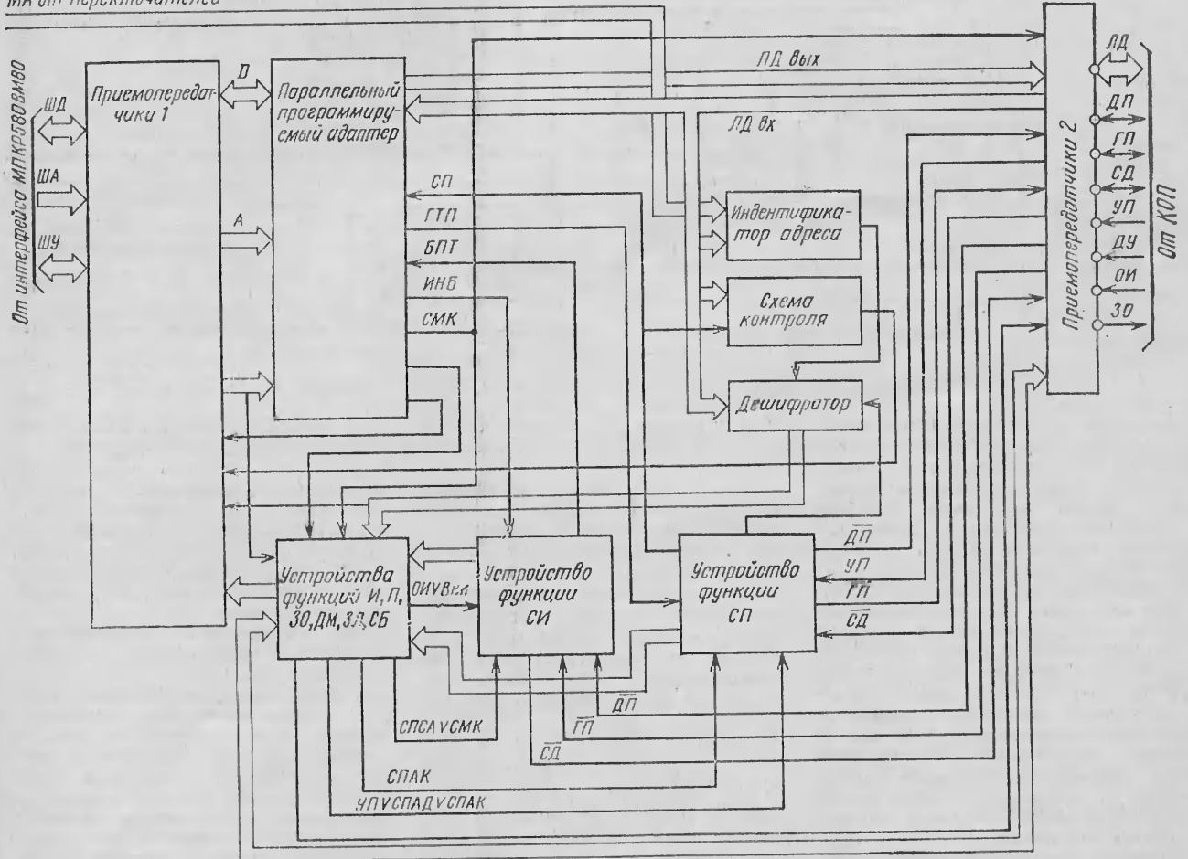
Рис. 2. Структурная схема интерфейса КОП:
