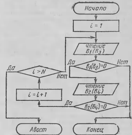
Рис. 4. Блок-схема программно управляемого асинхронного чтения
