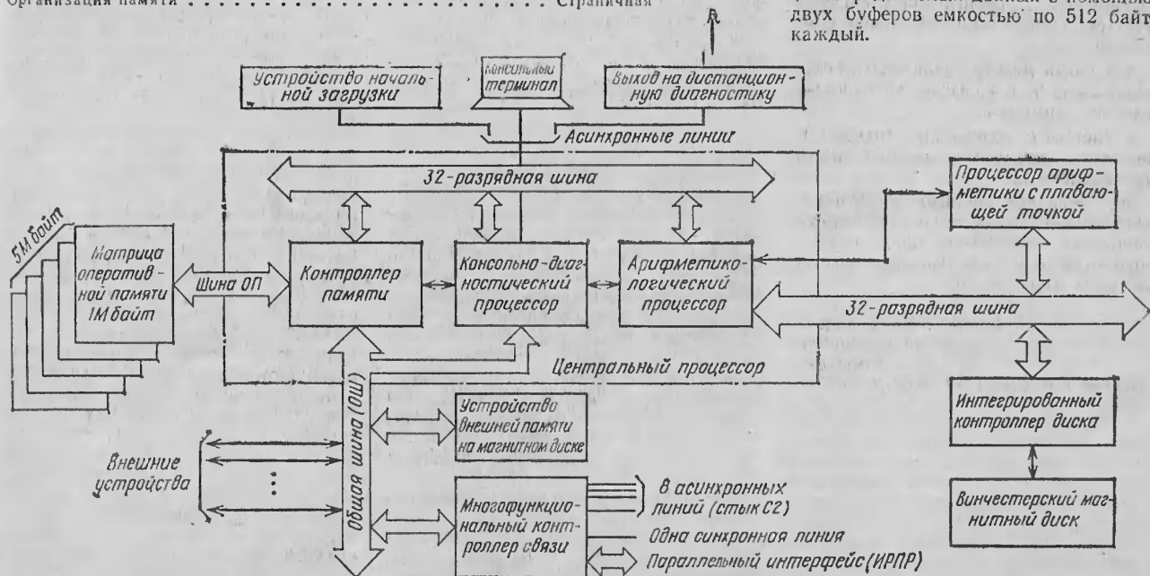
Структурная схема ВК СМ 1700
