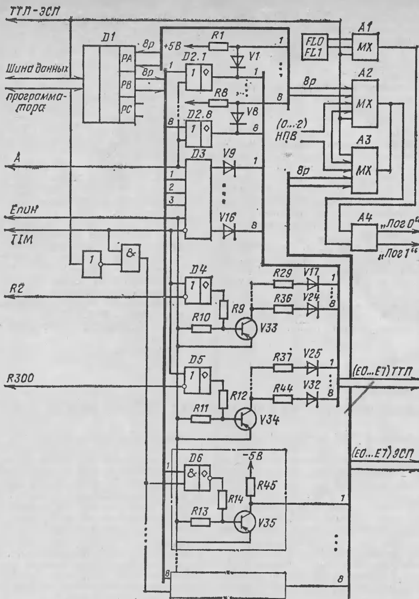
Рис. 3. Функциональная схема ключей данных
