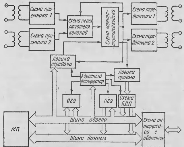
Рис. 2. Функциональная схема контроллера станции СЛК-СМ
