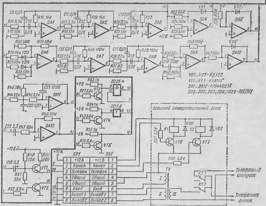
Рис. 2 (окончание). Принципиальная схема программно управляемого модема
