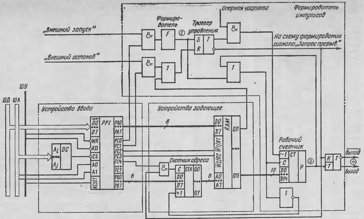
Рис. 2. Функциональная схема программно управляемого генератора импульсов
