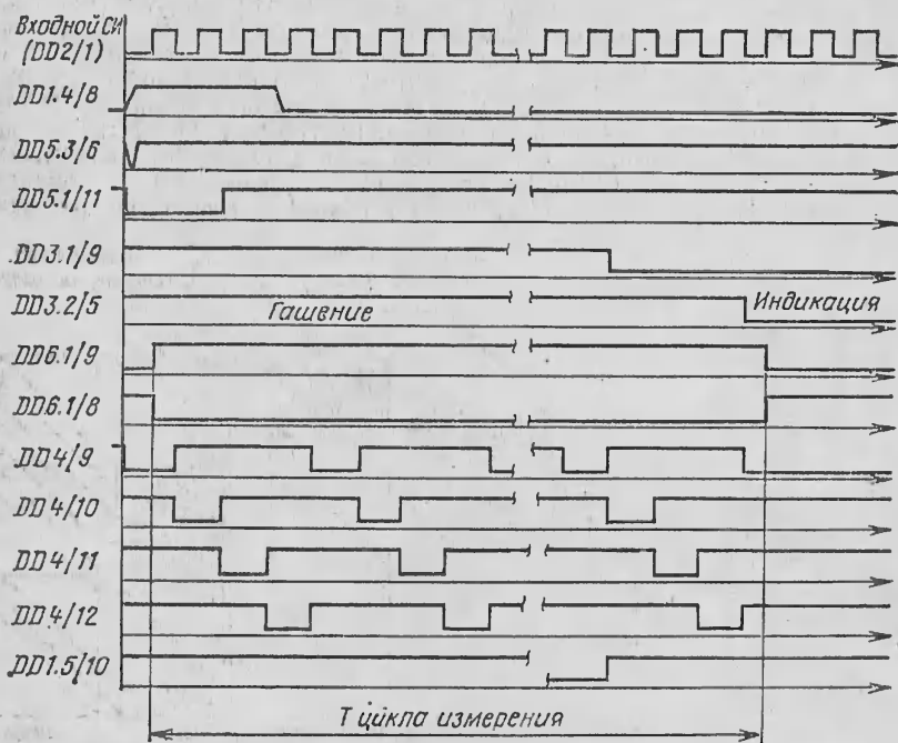
Рис. 4. Временные диаграммы сигнатурного анализатора
